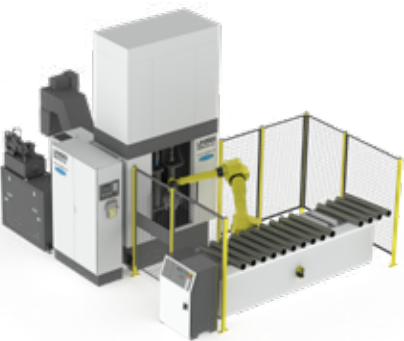
UNISIG SB100-2 Vertical skive burnish system with robotic automation Vertikales Schäl- und Glattwalzsystem mit Automatisierung
